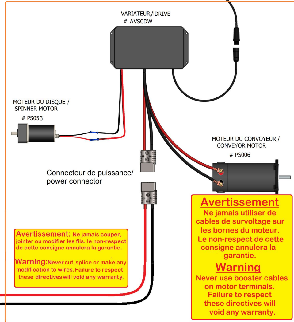
ARRIÈRE DE L'ÉPANDEUR / REAR OF THE SPREADER
