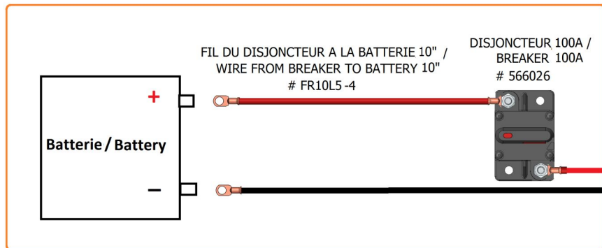
SOUS LE CAPOT / UNDER THE HOOD
